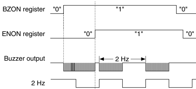
Fig. 4.12.3.2 2 Hz interval
